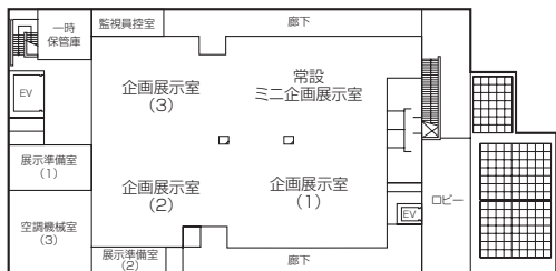
2階平面図
